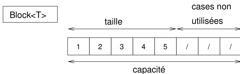
FIGURE 1 – Exemple d'une instance de Block<T> de taille 5 et de capacité 8
